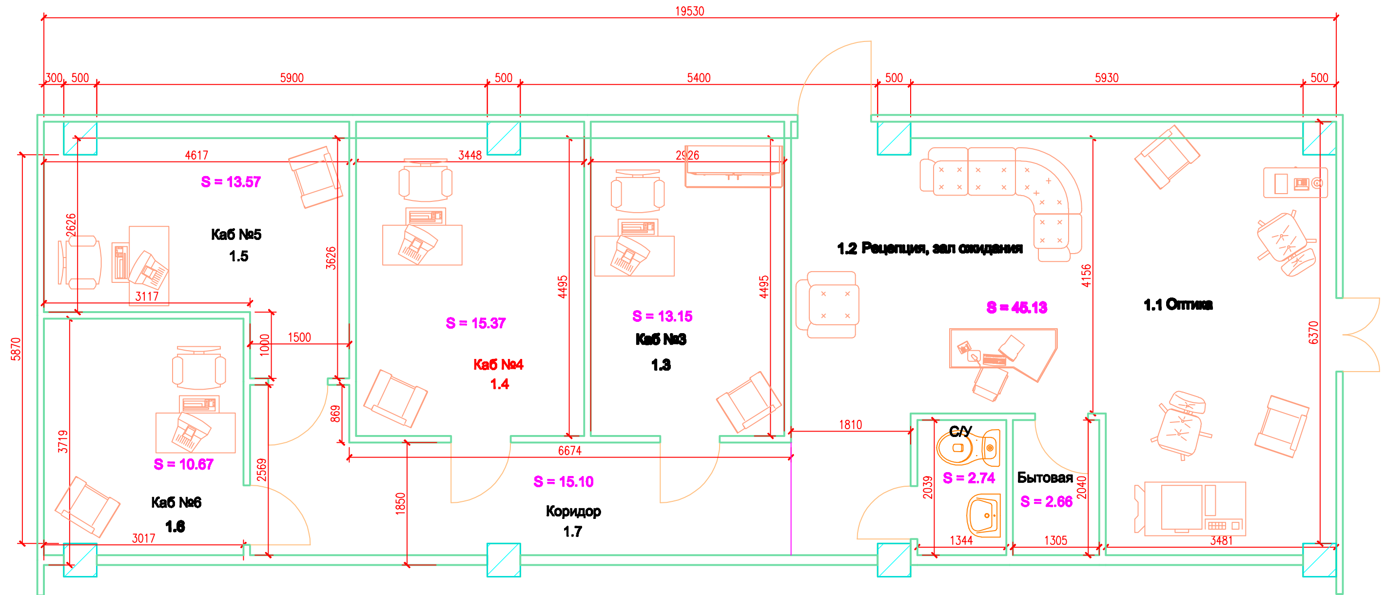
Експлікація приміщень 1-го поверху
